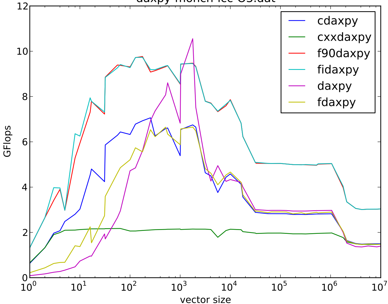
daxpy-monch-icc-O3.dat
